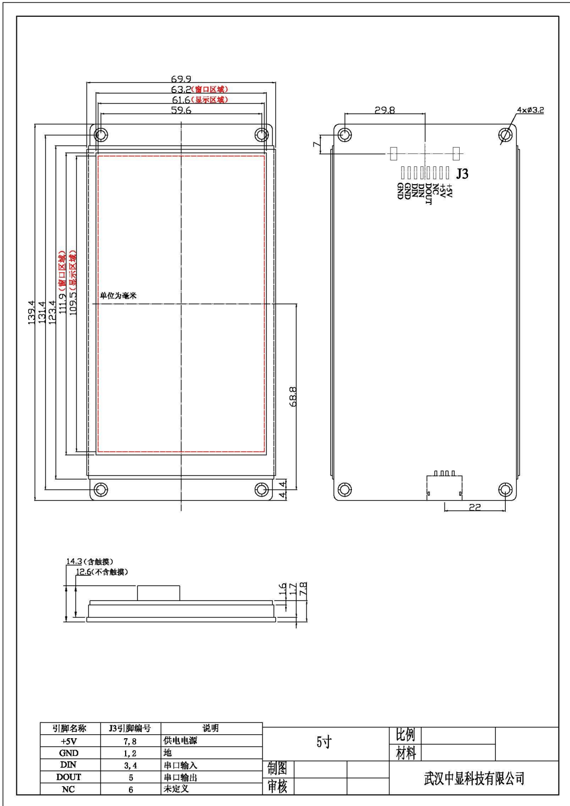
模块尺寸图
