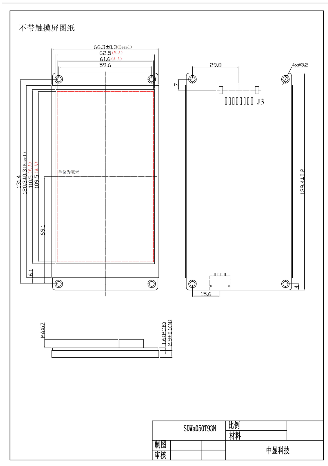
图 2 SDWa050T93N 尺寸图
