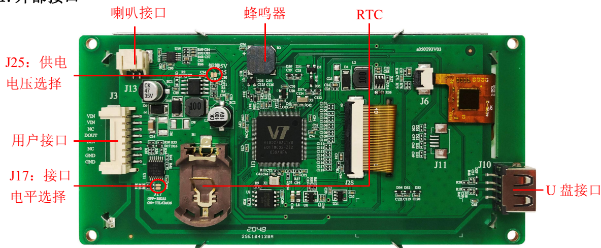
图 1 产品外观及硬件配置图
