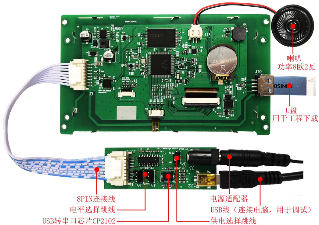
图 4 调试工具连接示意图
