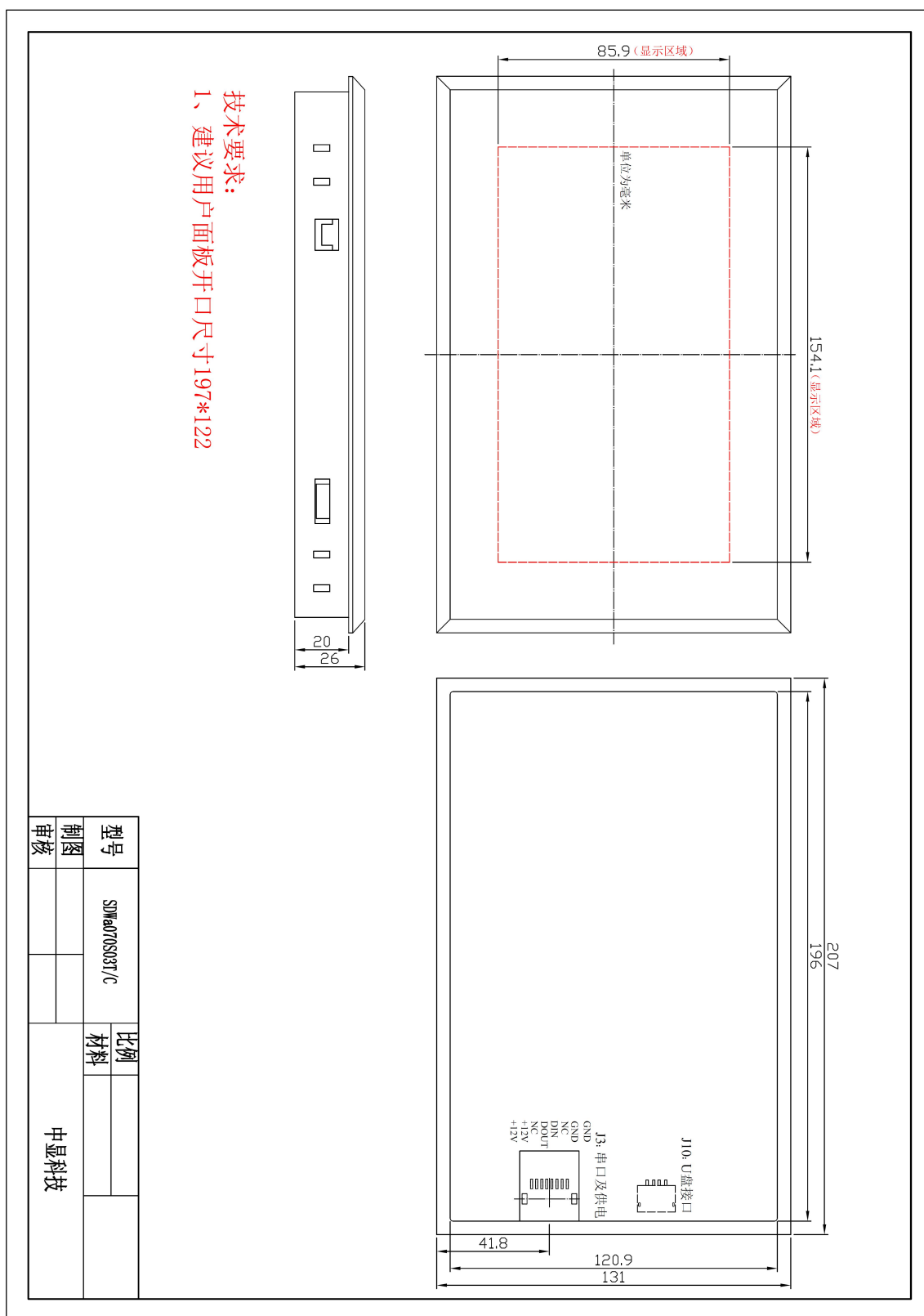
图 2 尺寸图
