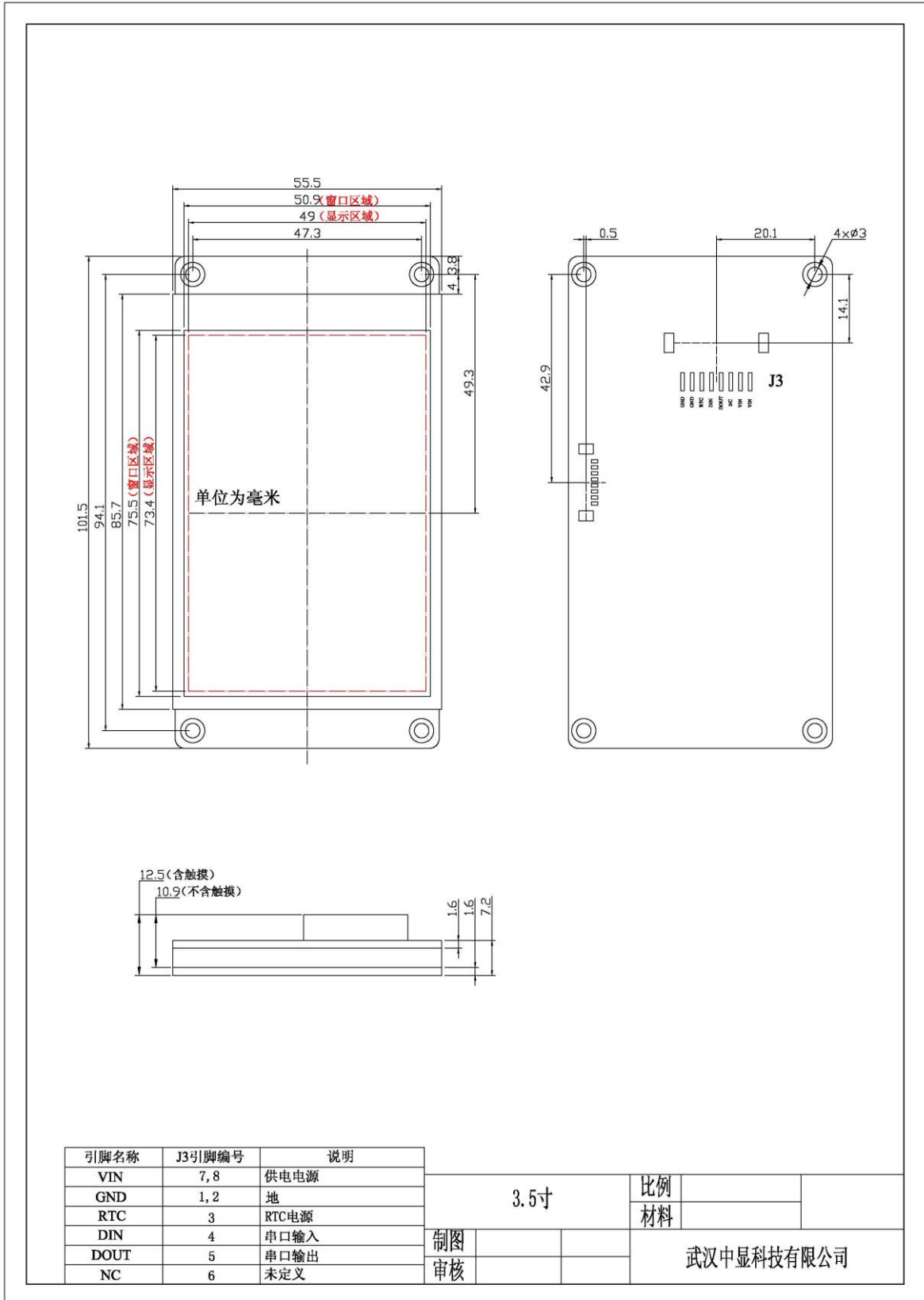
模块尺寸图
