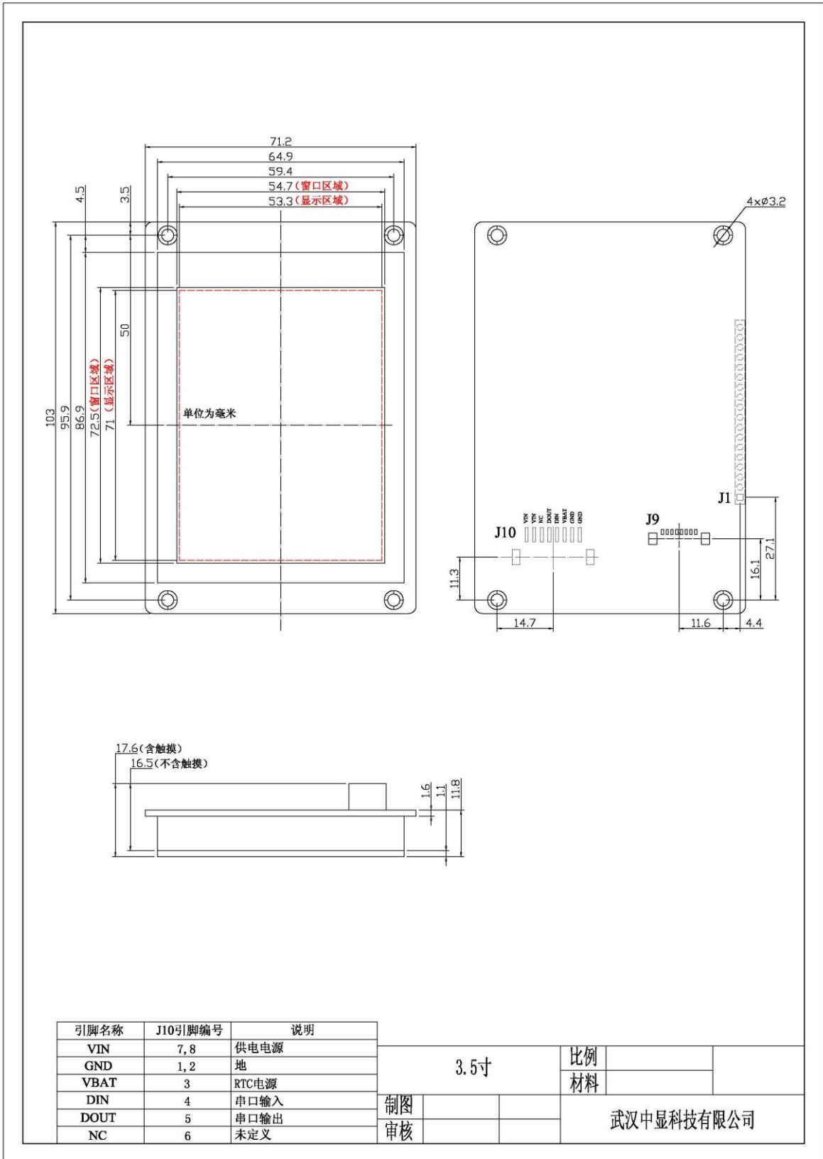
模块尺寸图
