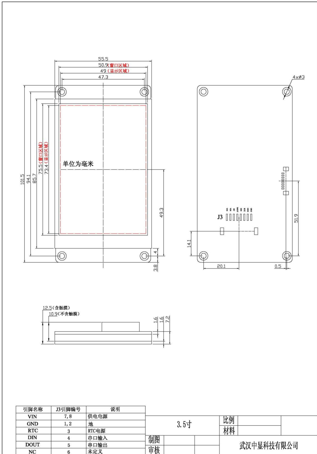
模块尺寸图
