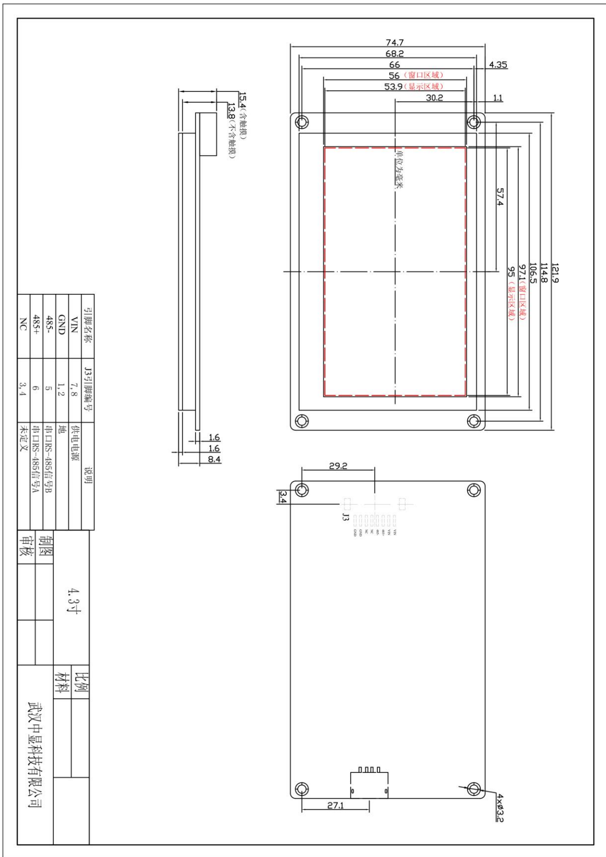
模块尺寸图
