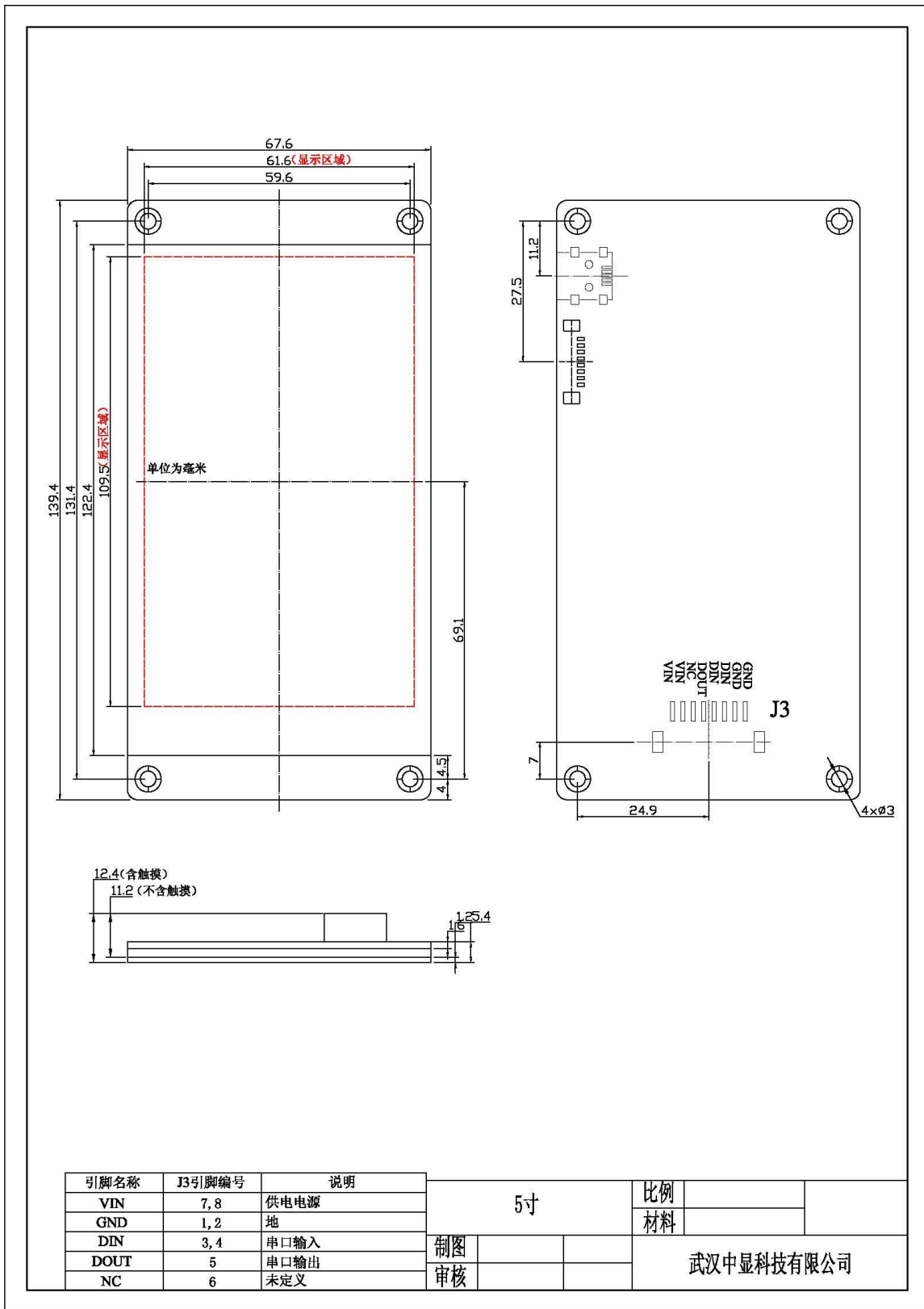
模块尺寸图
