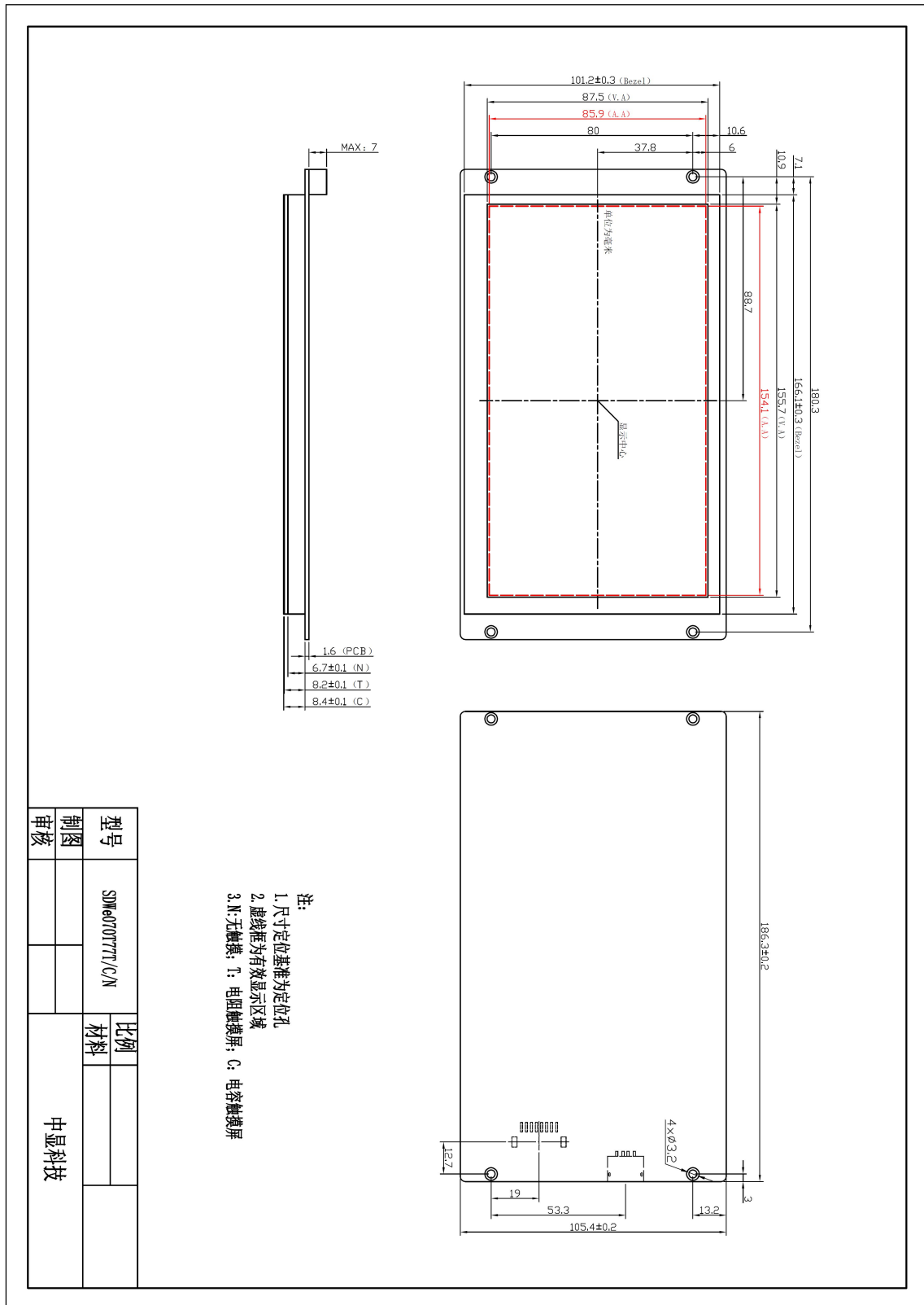
图2 尺寸图
