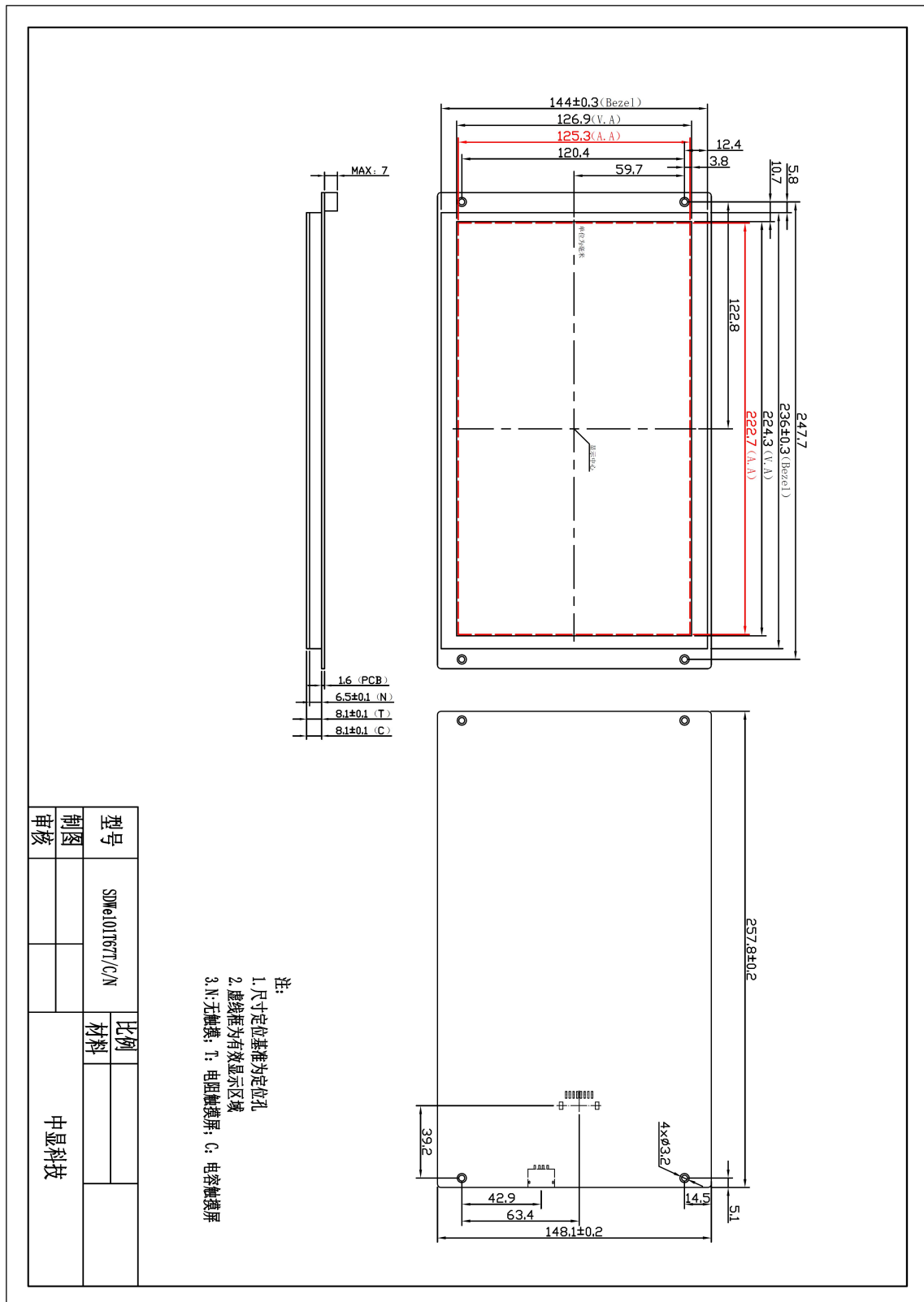
图 3 尺寸图
