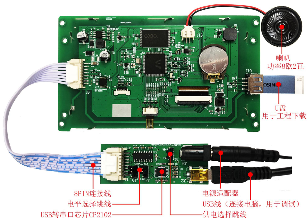
图 2 调试工具连接示意图
