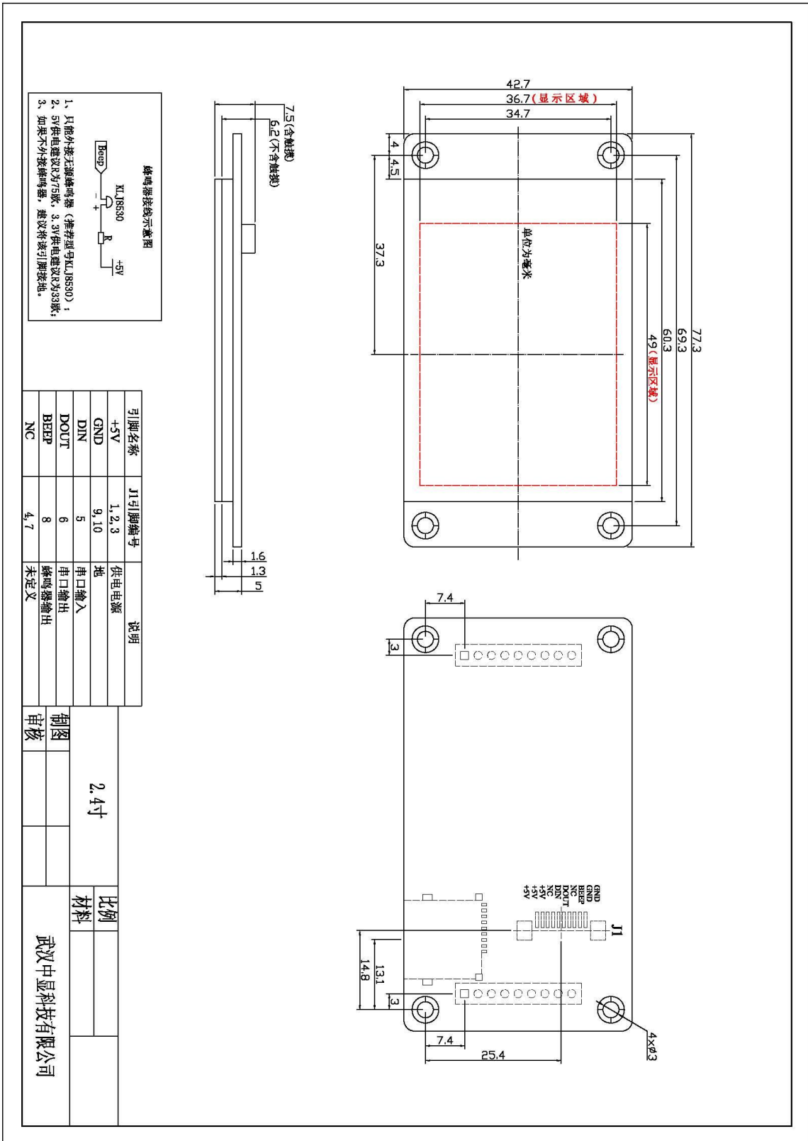
模块尺寸图
