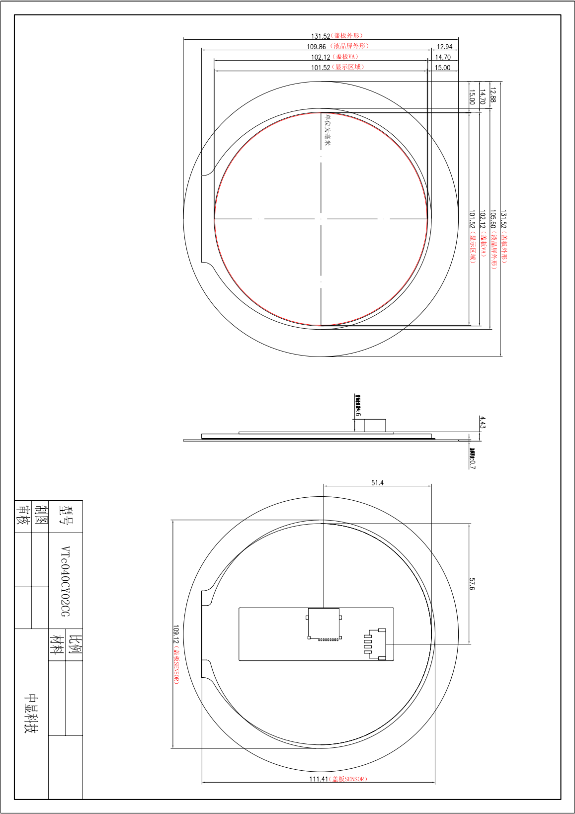
图 2 VTc040CY02CG 尺寸图
