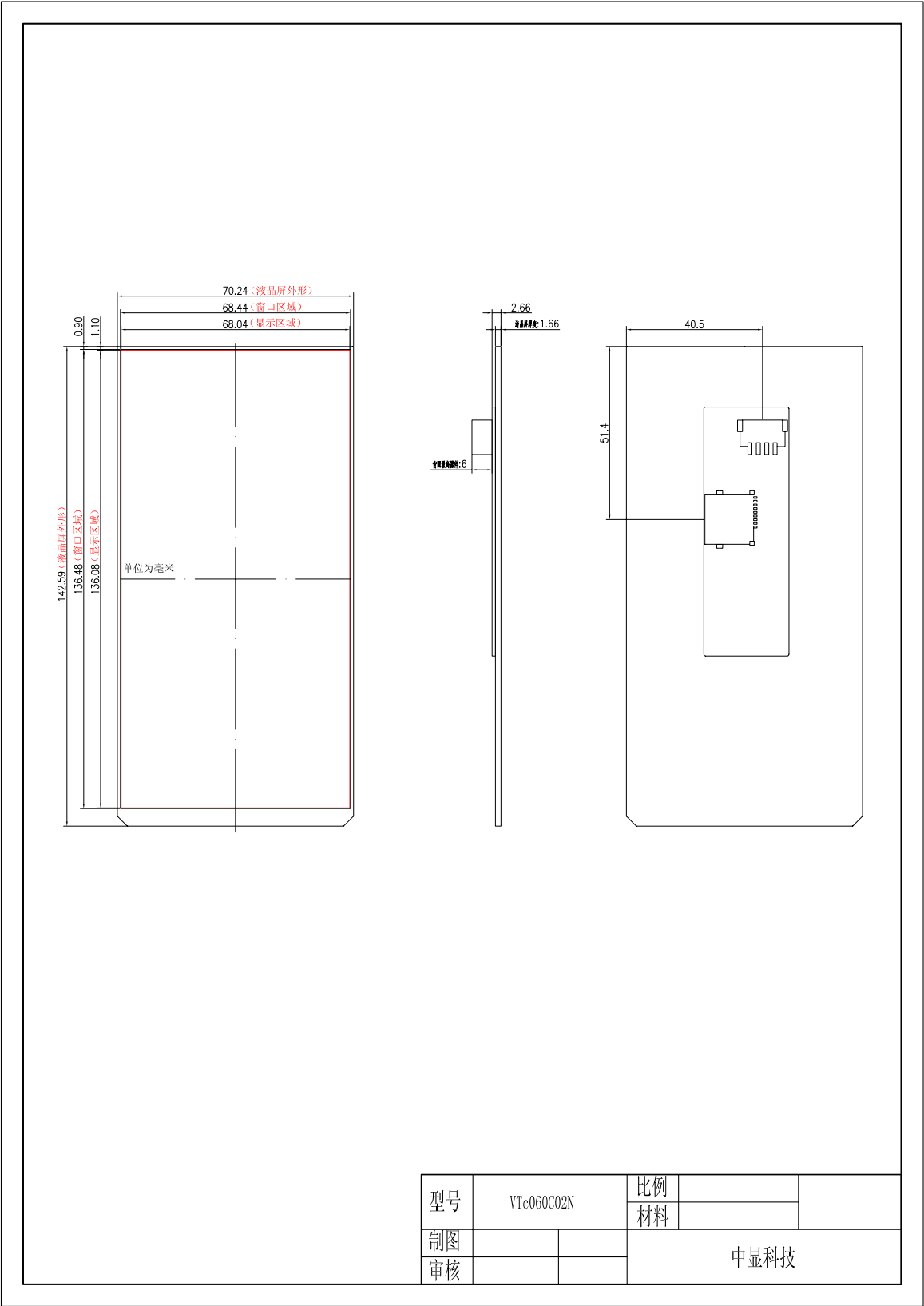
图 2 VTc060C02N 尺寸图
